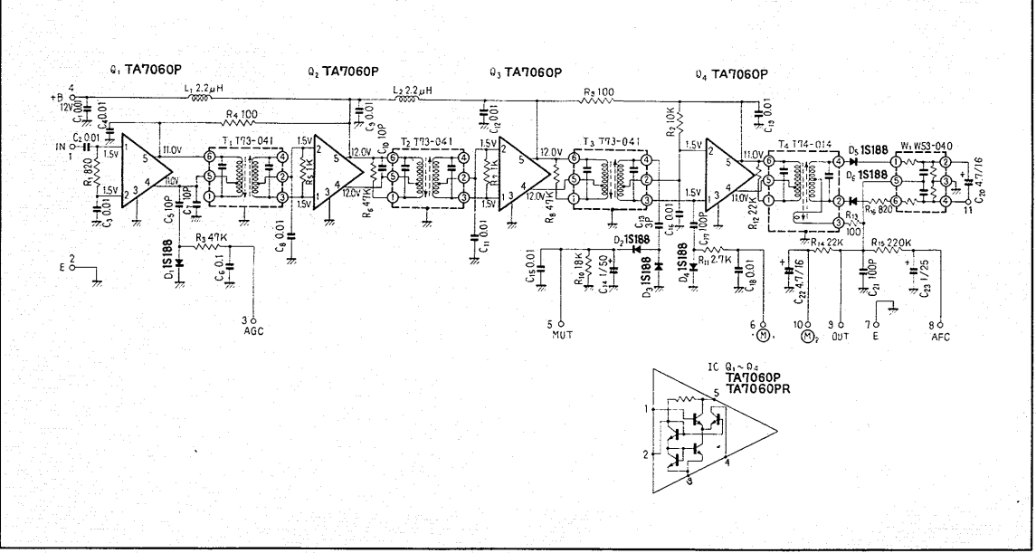
FM IF UNIT W12-032
